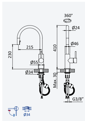
Sink mixer with swivel spout and pull out aerator - Ginger Mitigeur monocommande, bec mobile, avec mousseur extractible - Ginger
